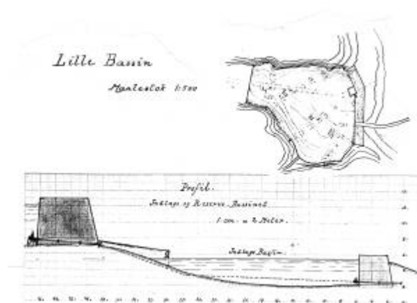
Plantegning og profil av Inntaksbassenget. Eigersund kommunes arkiv
